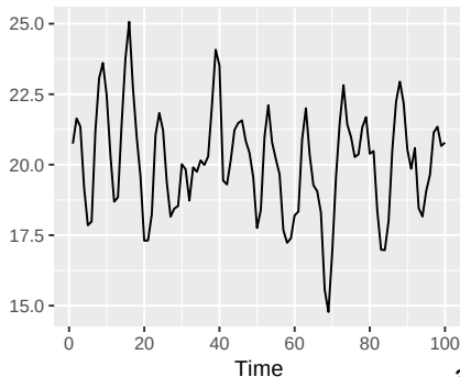
AR(2)
